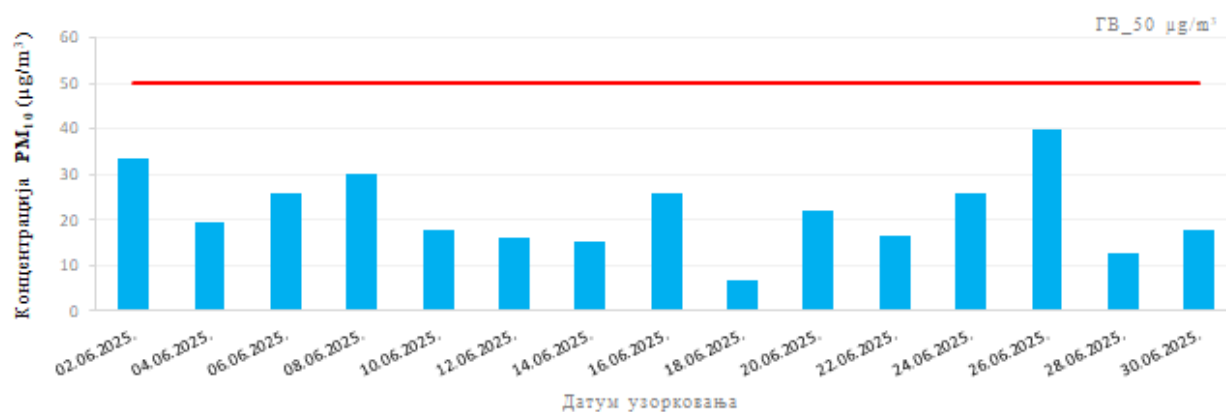
Слика 9. Резултати средњих дневних концентрација PM_{10} у ваздуху, на мм 1852-25_С2_Центар за културу у Смедереву, у периоду јун 2025. године
