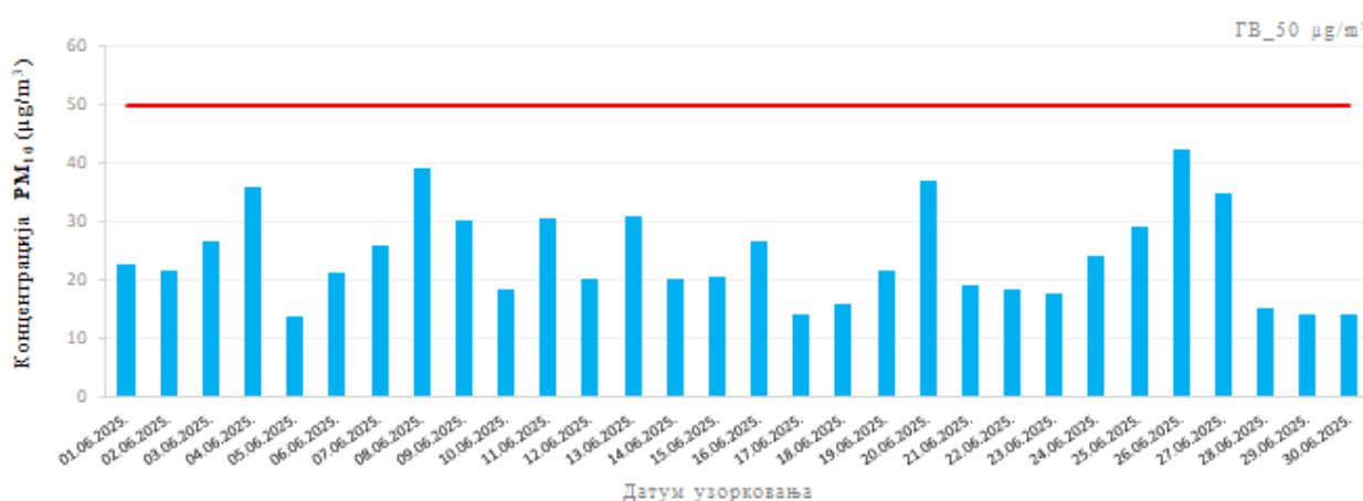
Слика 8. Резултати средњих дневних концентрација PM_{10} у ваздуху, на мм 1852-25_С1_Раља_домаћинство Ђорђевић, у периоду јун 2025. године
