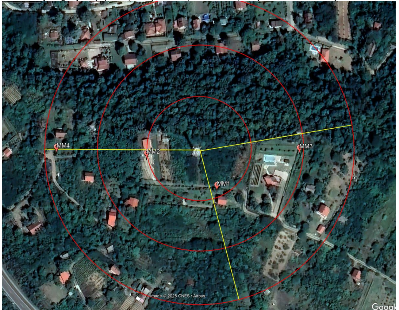
Slika 4: Prikaz Mernih Mesta u lokalnoj zoni oko planirane BS BA1536_01 SD_Jugovo
