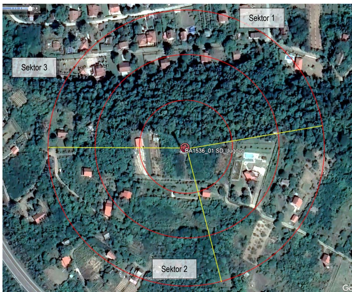
Slika 2.5 Pravci zračenja antenskog sistema predmetne bazne stanice
